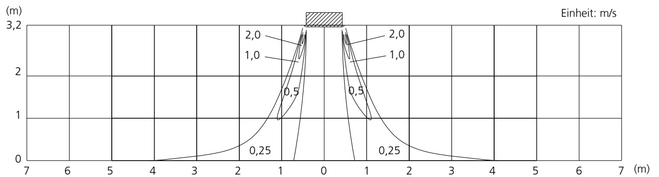
Seitenansicht Vertikale Lamellen : Position 4
