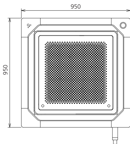
Unteransicht (Ansicht A)
