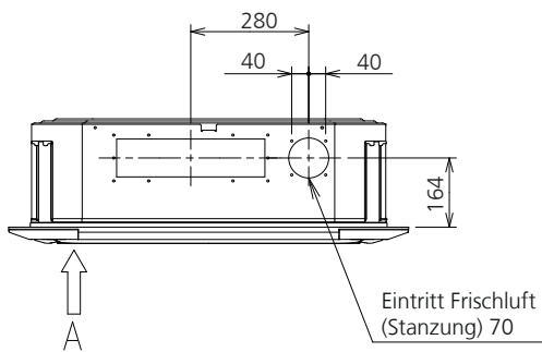
Ansicht B
