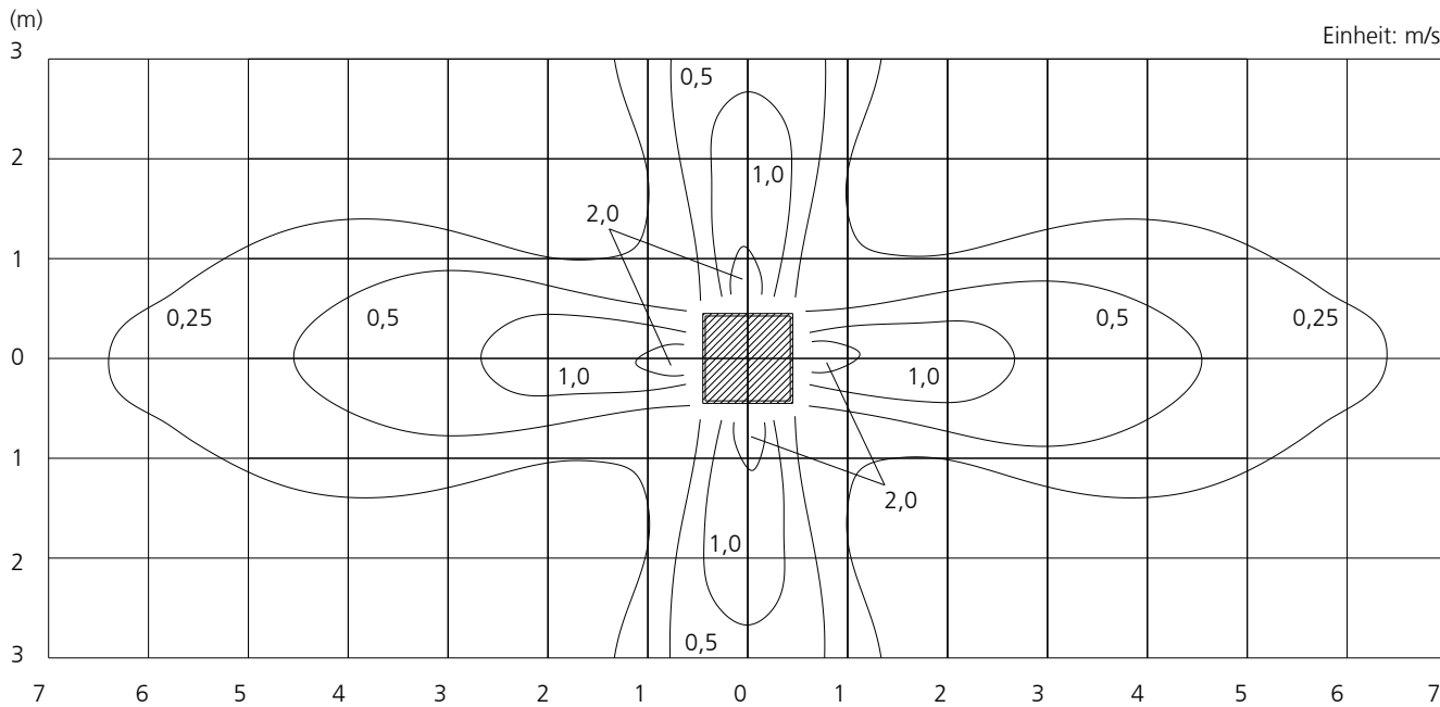
Draufsicht Vertikale Lamellen : Position 1
