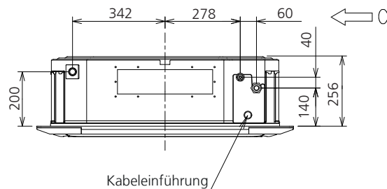
Seitenansicht
