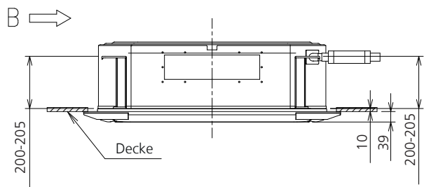
Seitenansicht
