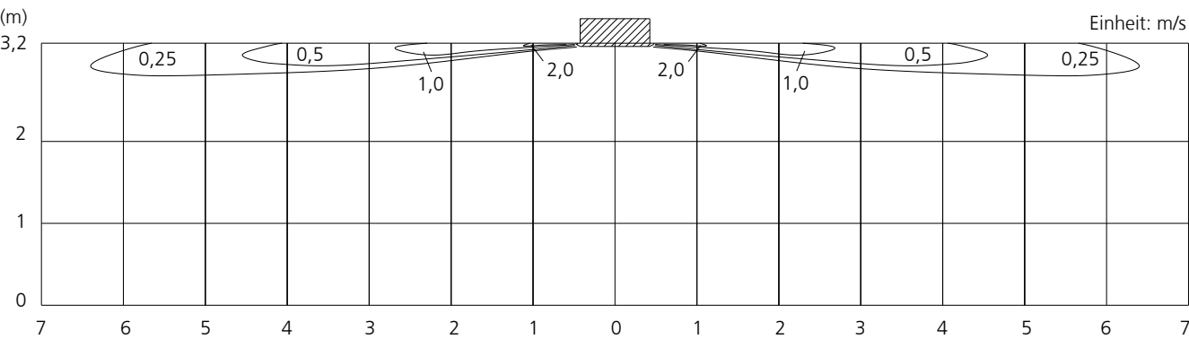
Seitenansicht Vertikale Lamellen : Position 1
