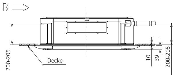
Seitenansicht
