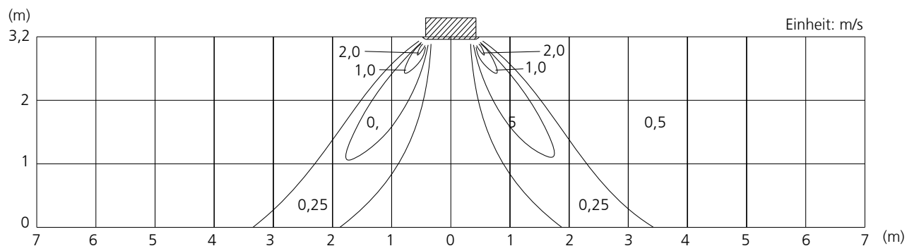
Seitenansicht Vertikale Lamellen : Position 2
