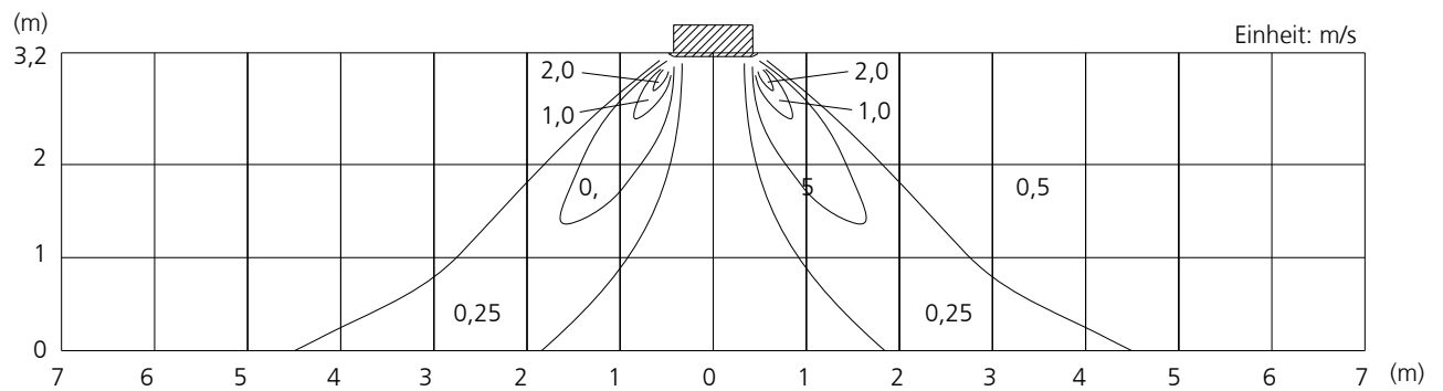
Seitenansicht Vertikale Lamellen : Position 2
