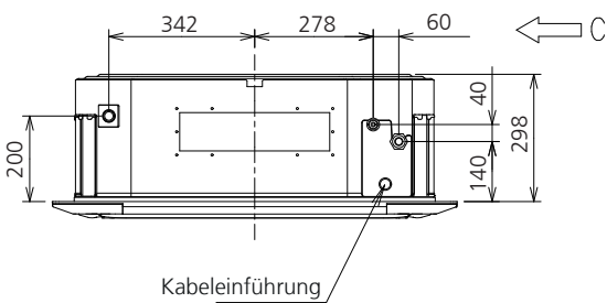
Seitenansicht
