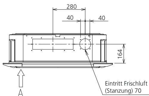
Ansicht B
