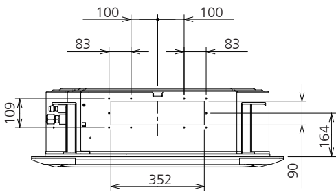
Seitenansicht
