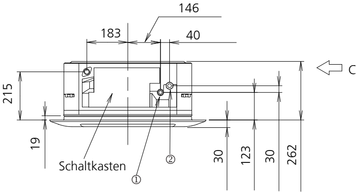
Seitenansicht
