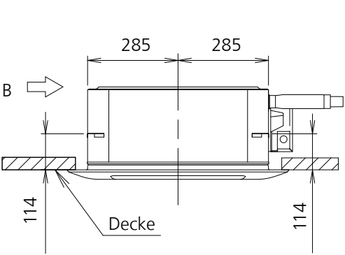
Seitenansicht
