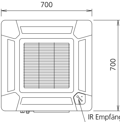
Unteransicht (Ansicht A)
