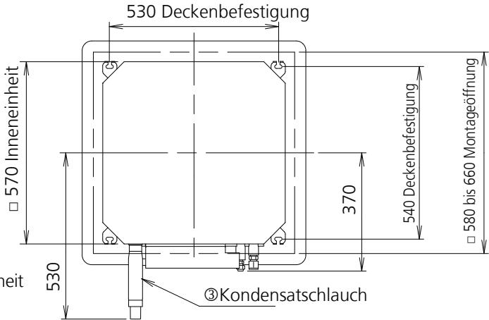
Draufsicht
