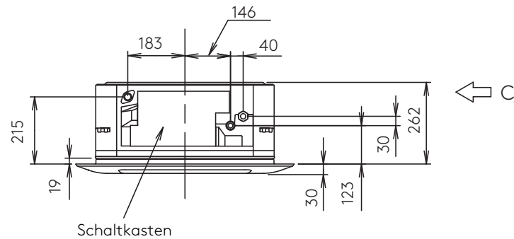
Seitenansicht
