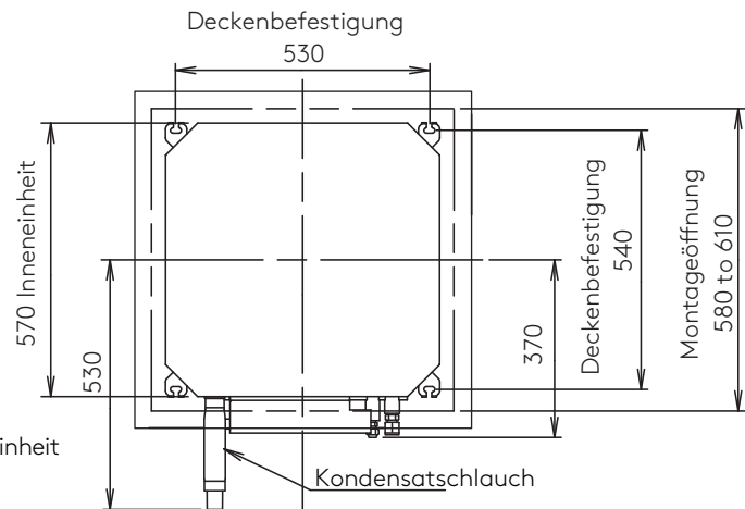
Draufsicht
