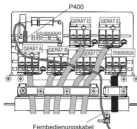
Anschluss zentrale Fernbedienung
