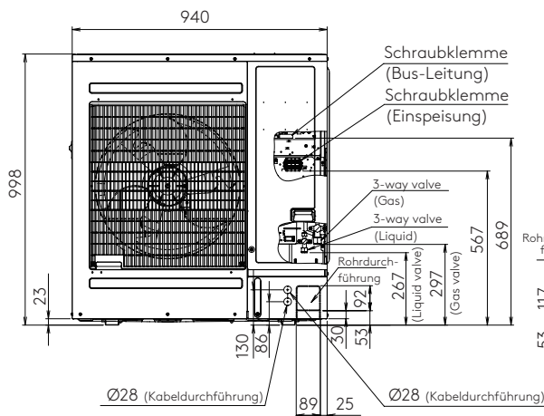
Frontansicht
