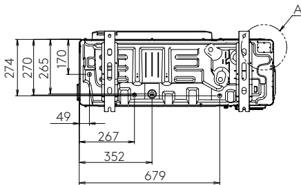
Untersicht
