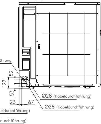
Rückansicht
