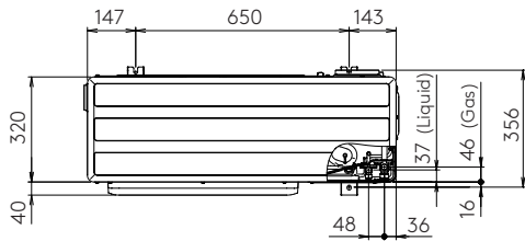
Draufsicht
