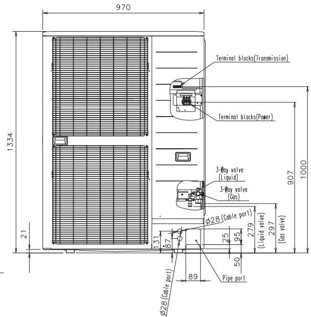
Frontansicht
