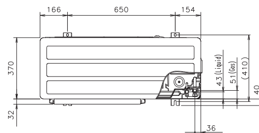
Draufansicht
