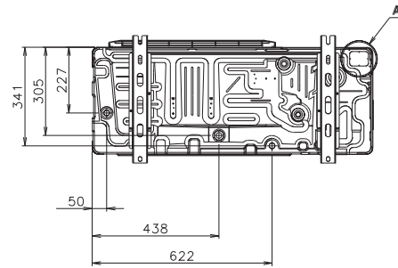
Unteransicht
